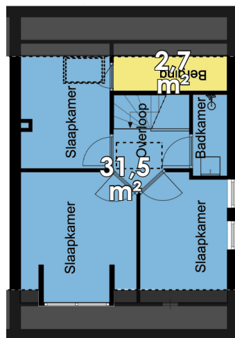
1e Verdieping
