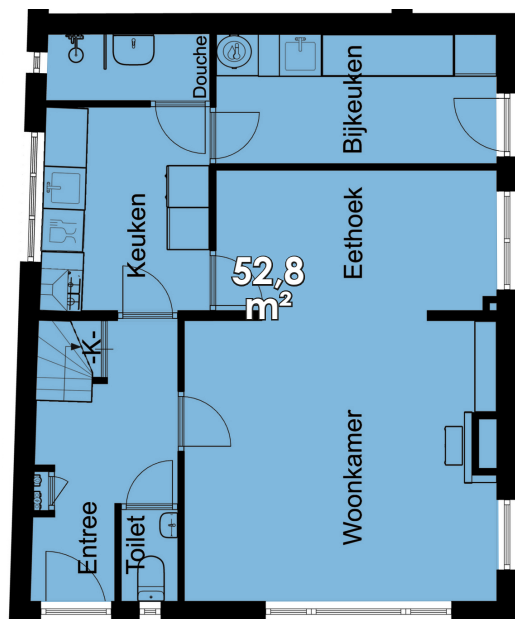
Begane grond
